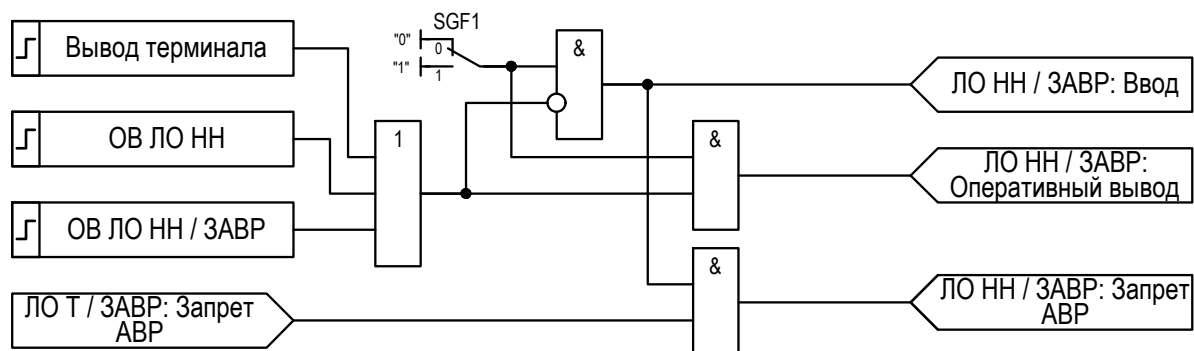
Рисунок 2.25 – Функциональная схема «Запрет АВР»
