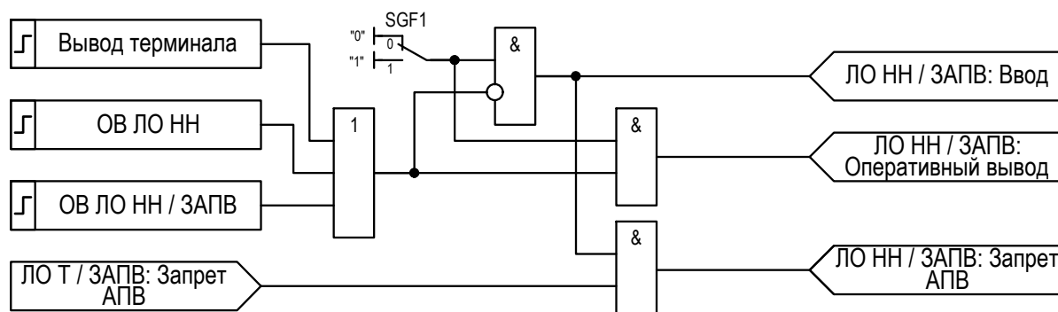
Рисунок 2.24 – Функциональная схема «Запрет АПВ»
