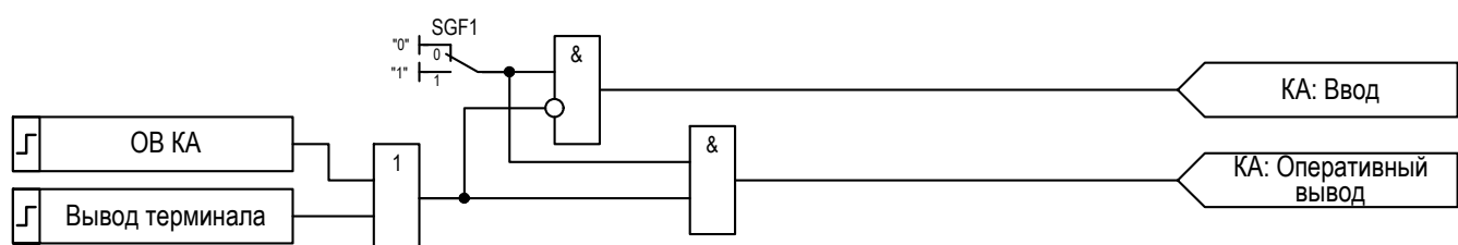
Рисунок 2.32 – Логика управления режимами функционального блока «КА»
