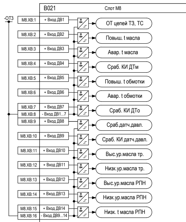
Рисунок Г.3 – Подключение дискретных входов и выходов к внутренним сигналам алгоритмов для блоков в слотах M6-M8
