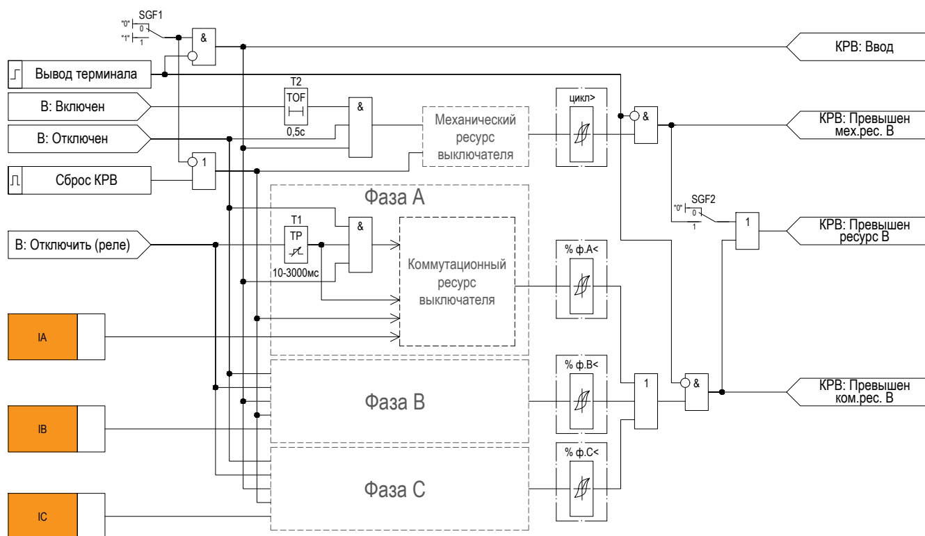
Рисунок 2.27 – Функциональная схема «КРВ»
