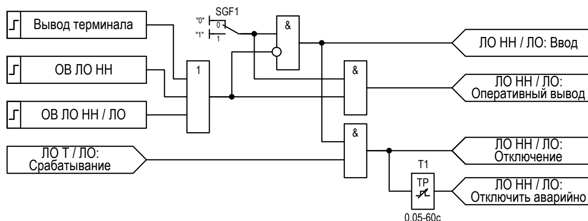
Рисунок 2.23 – Функциональная схема «ЛО»
