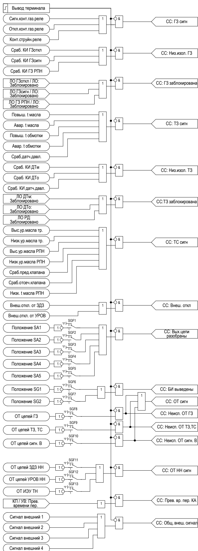
Рисунок 2.34 – Функциональная схема «СС»
