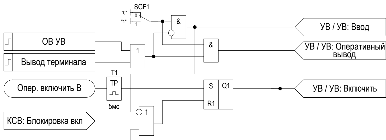
Рисунок 2.31 – Функциональная схема «УВ»
