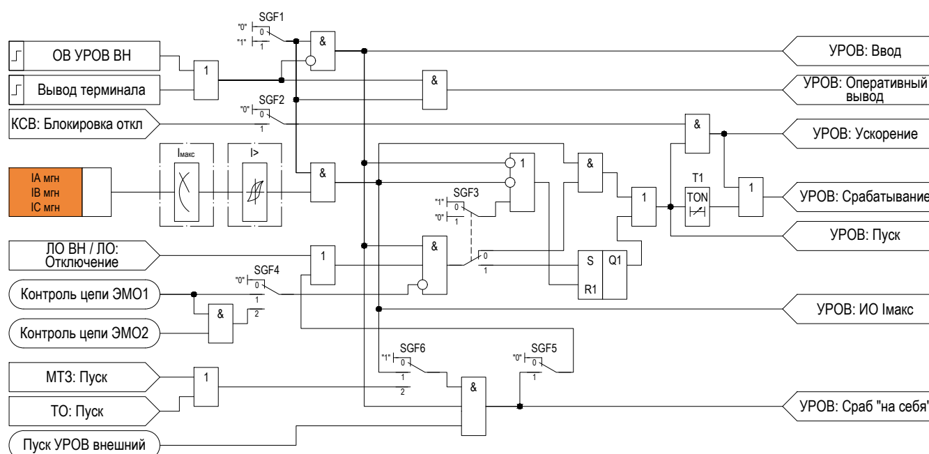
Рисунок 2.26 – Функциональная схема «УРОВ»
