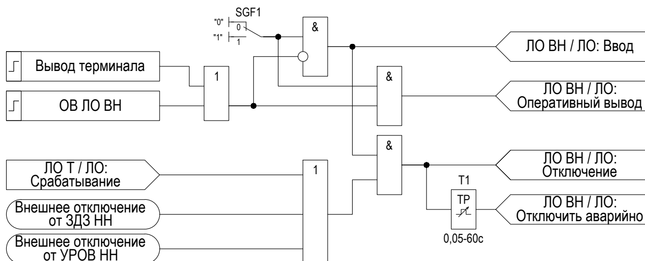
Рисунок 2.22 – Функциональная схема «ЛО»
