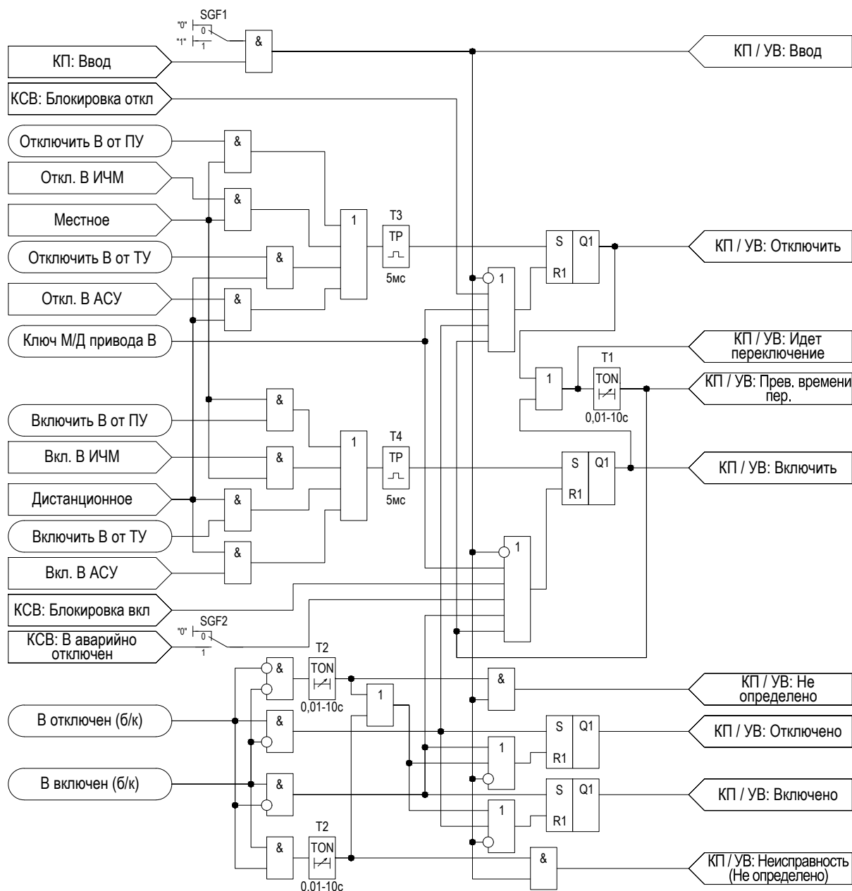
Рисунок 2.30 – Функциональная схема «УВ»
